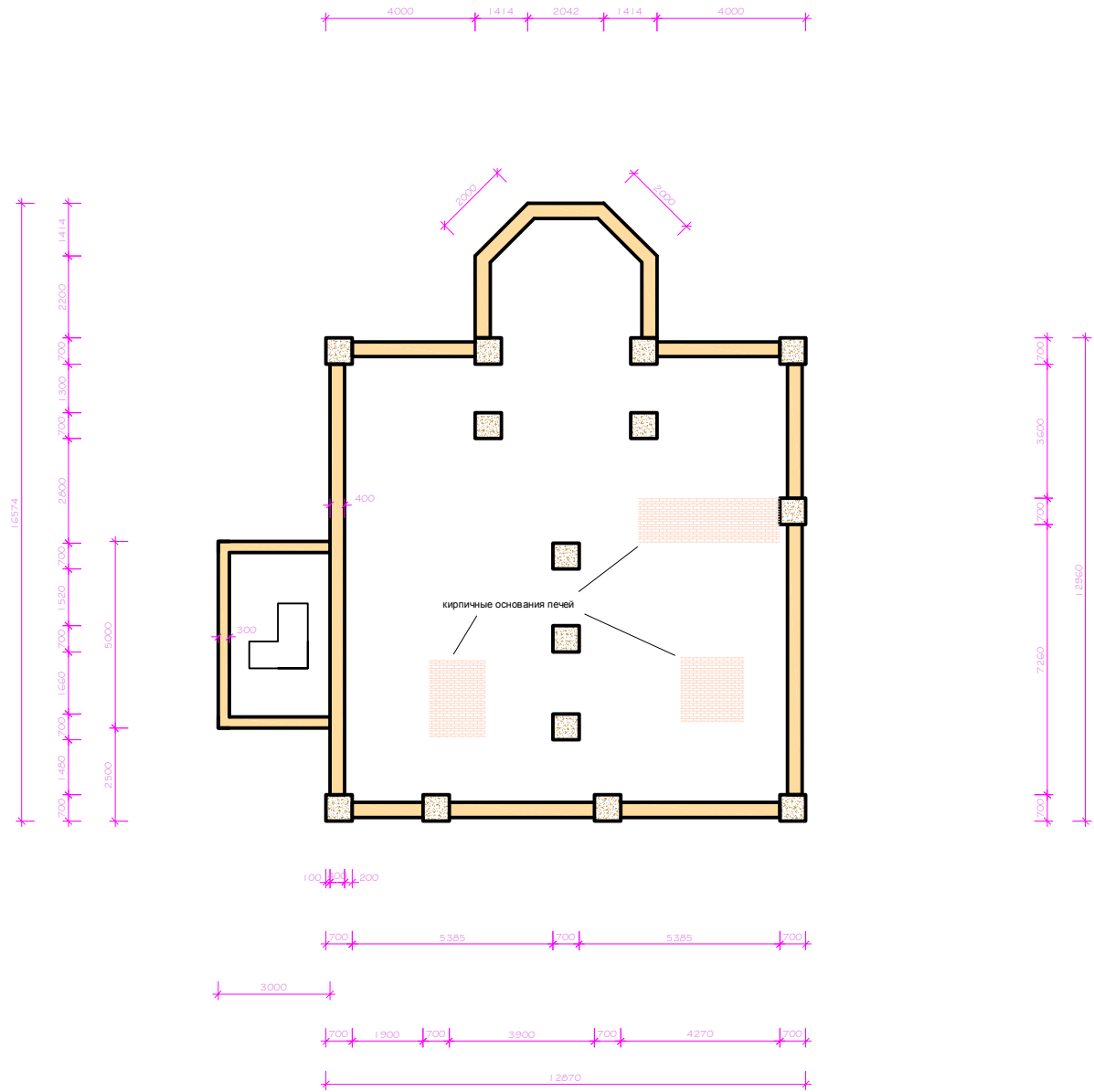
План фундамента гостиницы Куулушона в п . Вырица угол ул . Крайняя (1-Мая) и Сиверского шоссе .
